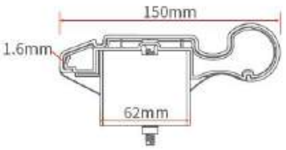
HS-676树脂 防护扶手 产品材质: 热塑型高分子材料+铝镁合金 整体厚度: 70mm 产品规格: 4000mm*150mm
